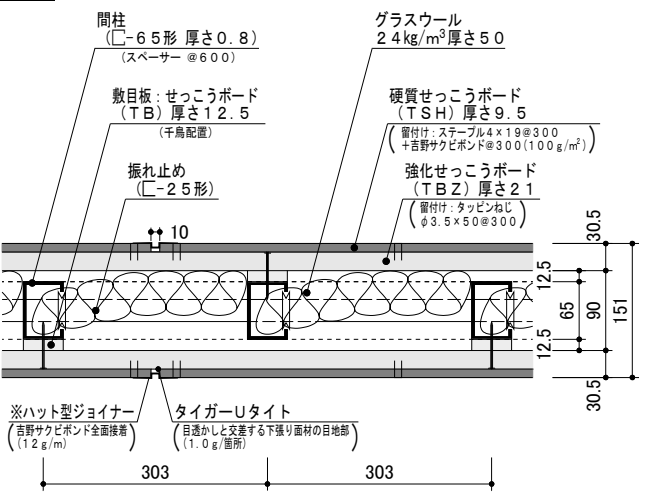
水平断面図
