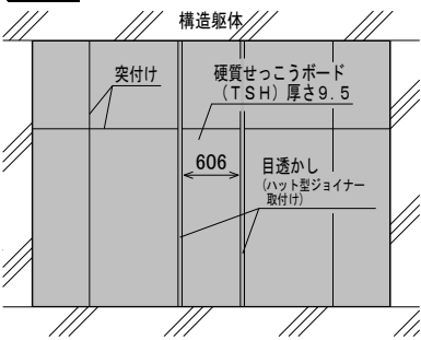
正面図
