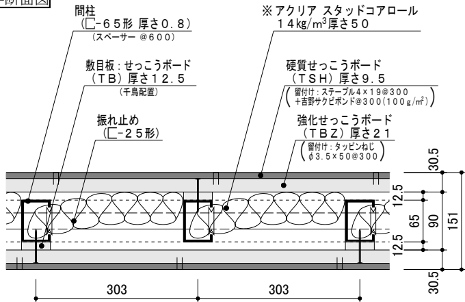
水平断面図
